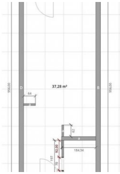
Grundriss
